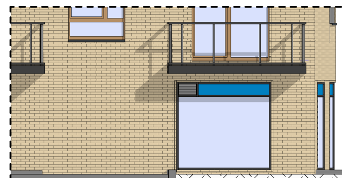
2 ELEWACJA WSCHODNIA
